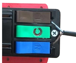
2 WIRE
